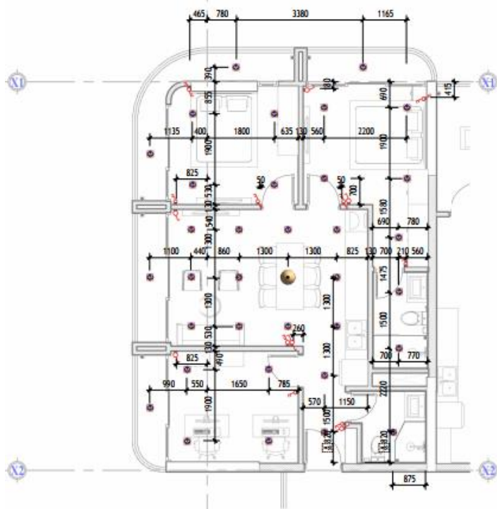
1 MẶT BẰNG Ô CẮM - BÓNG ĐIỆN 1 : 80
