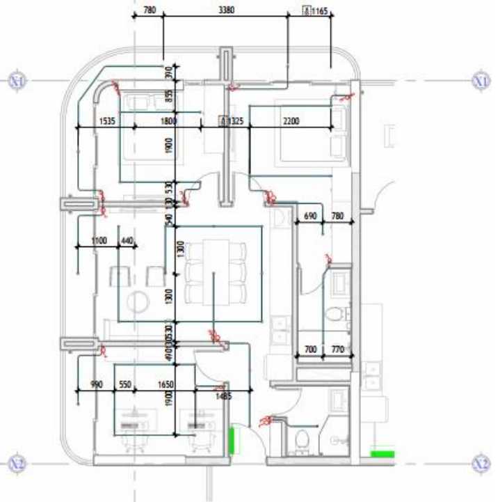
2 MẶT BẰNG ỐNG DẪN - BOX ĐIỆN 1 : 80
