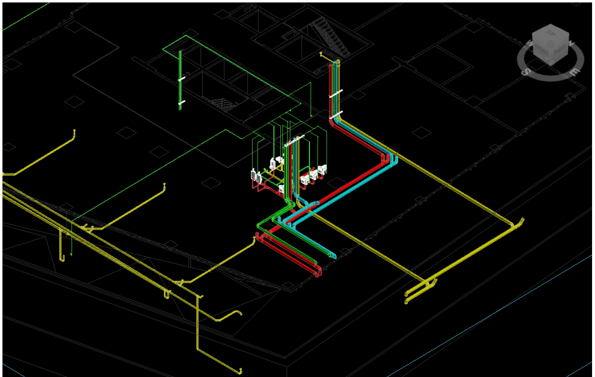
Dựng hình ống thoát nước thải WC tầng gom về bể xử lý.
