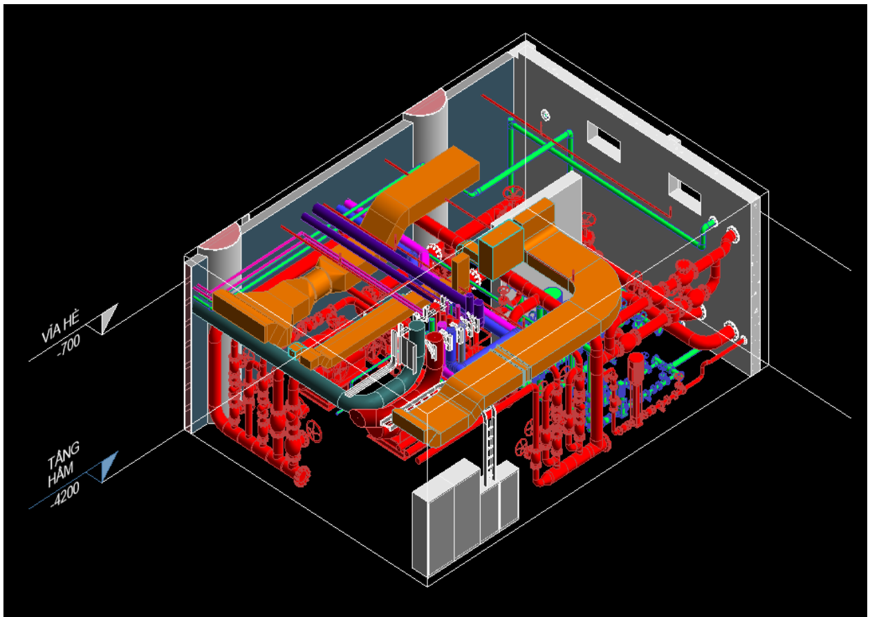
Combine Hệ thống MEPF phòng bơm Chữa cháy dự án L'avenir Quy Nhơn.
