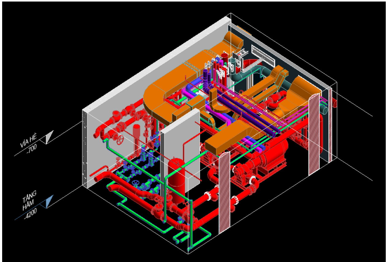
Combine Hệ thống MEPF phòng bơm Chữa cháy dự án L'avenir Quy Nhơn.
