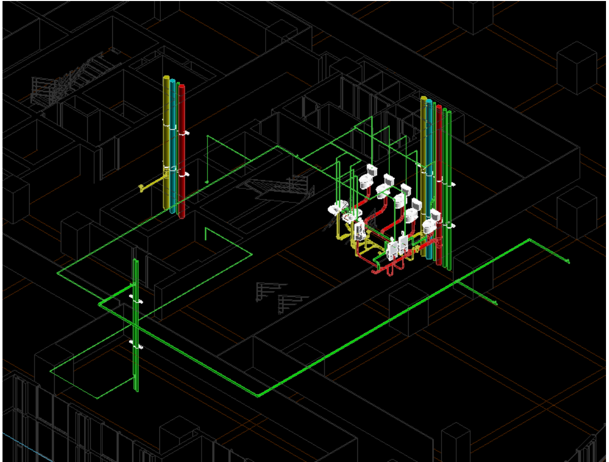
Dựng hình hệ thống ống cấp nước, thoát nước thải WC điển hình.
