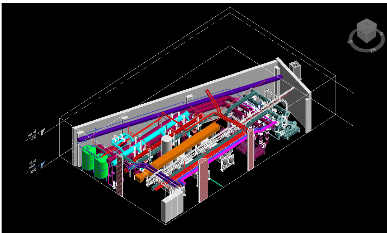
Combine Hệ thống MEPF phòng máy Chiller dự án L'avenir Quy Nhơn.
