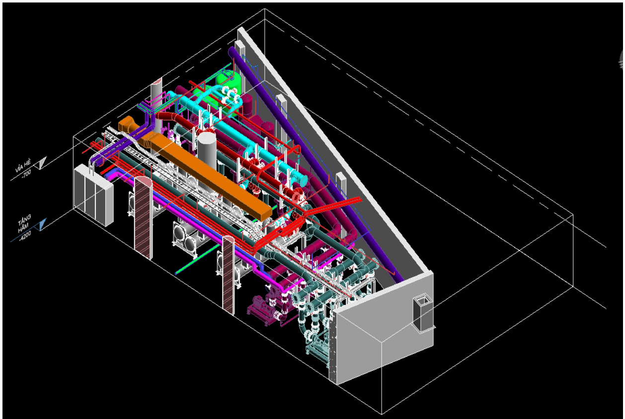
Combine Hệ thống MEPF phòng máy Chiller dự án L'avenir Quy Nhơn.
